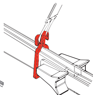
ÉTAPE 3 : Passer les boucles des extrémités de la sangle dans la partie haute des crochets des klipskis
