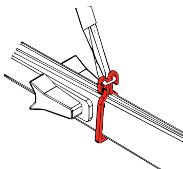
ÉTAPE 3 : Passer les boucles des extrémités de la sangle dans la partie haute des crochets des klipskis
