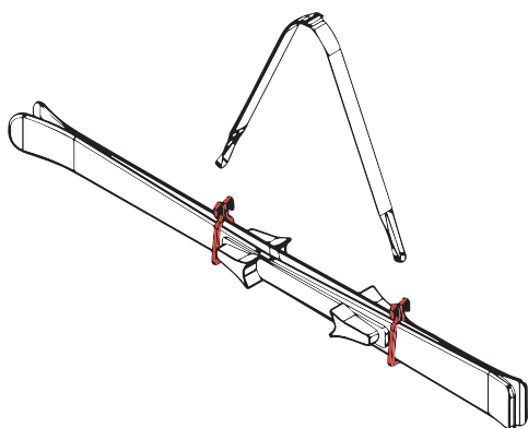
ÉTAPE 3 : Passer les boucles des extrémités de la sangle dans la partie haute des crochets des klipskis
